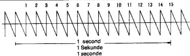
Abb. 1 15Hz-Sägezahnwelle
